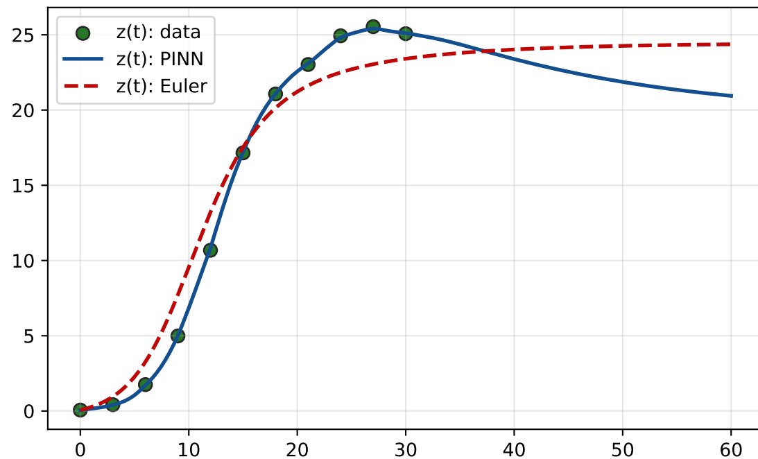
z(t): Ethanol
