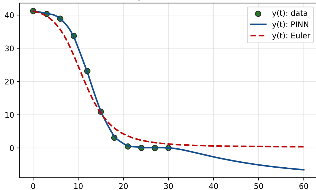
y(t): Fructose
